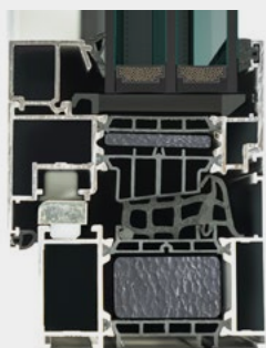
2-zložkové centrálné tesnenie
